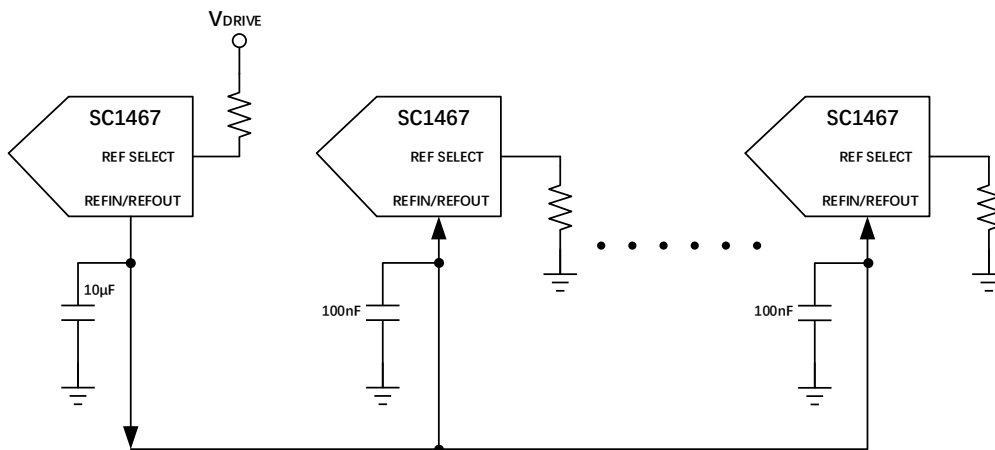
图 10 内部基准驱动多个 SC1467 REFIN 引脚
