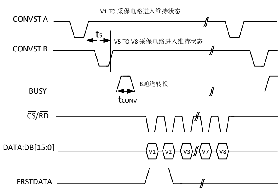
图 12 SC1467 使用独立的 CONVST A 和 CONVST B 信号时对通道集进行同步采样（并行模式）
