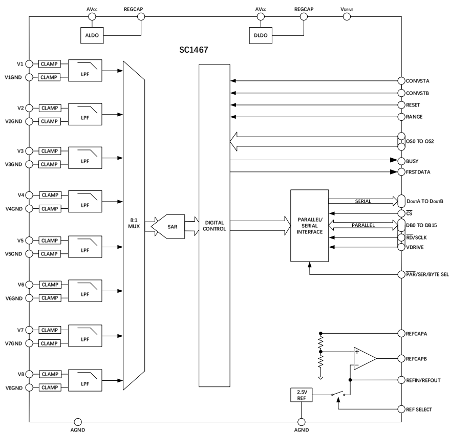
图 1 SC1467 芯片模块示意图
