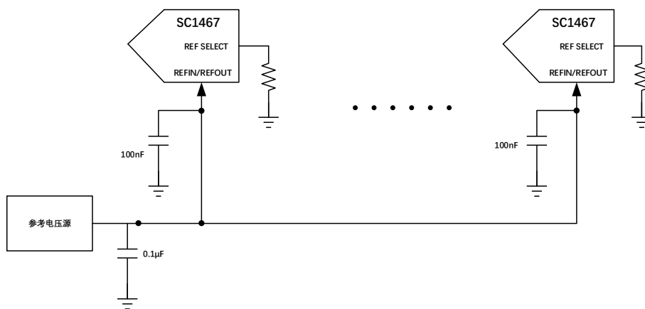
图 9 单个外部基准驱动多个 SC1467 REFIN 引脚
