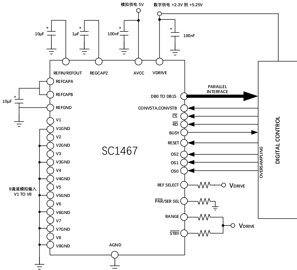
图 11 SC1467 典型连接关系图
