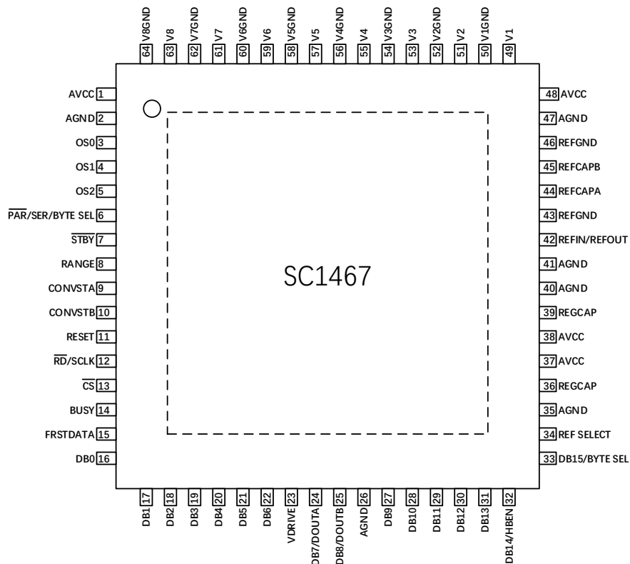
图 8 8 通道 SC1467 管脚（焊盘）配置（俯视图）
