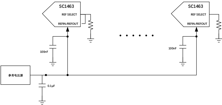
图 9 单个外部基准驱动多个 SC1463 REFIN 引脚
