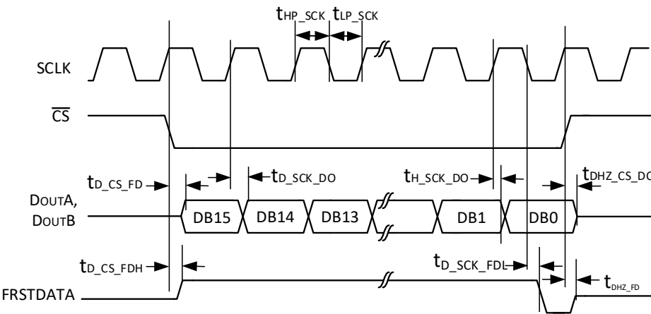
图 6 串行时序图，ADC 读取模式（通道 1）
