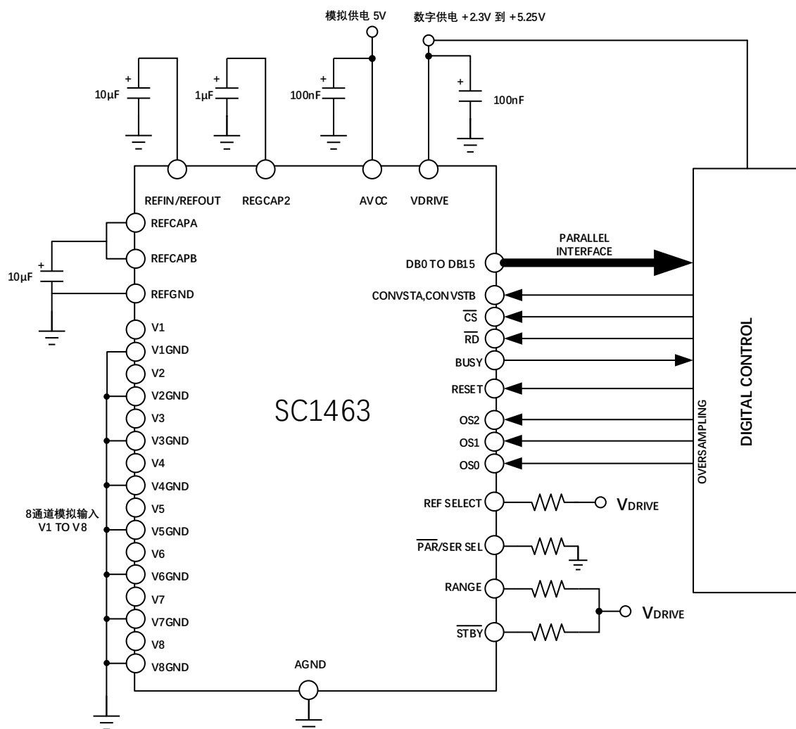
图 11 SC1463 典型连接关系图
