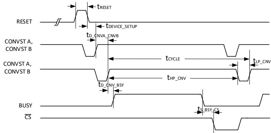
图 2 转换时序图，转换后读入数据
