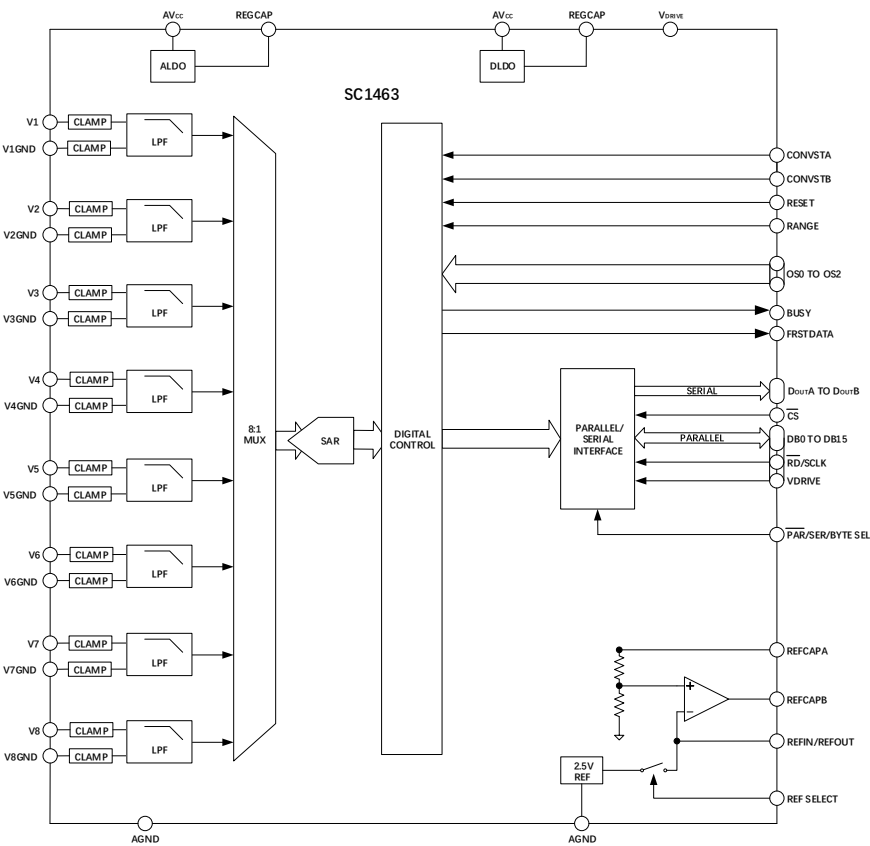
图 1 SC1463 芯片模块示意图
