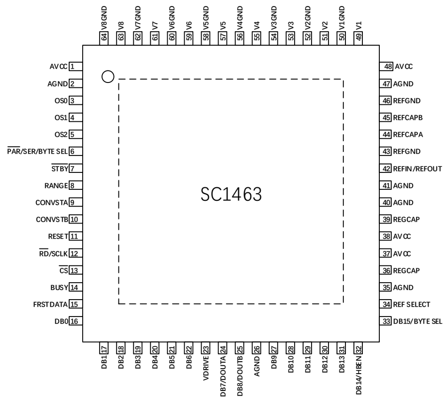
图 8 8 通道 SC1463 管脚（焊盘）配置（俯视图）
