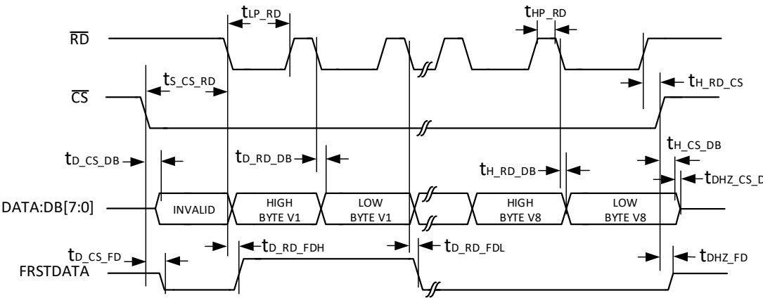
图 7 串行接口时序图，字节模式读操作
