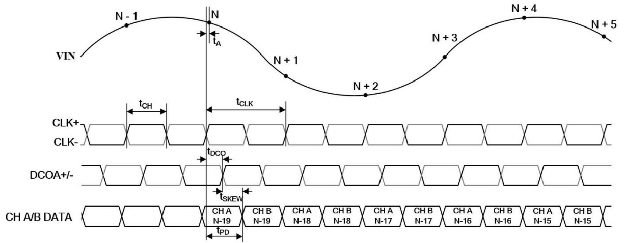
图 4 LVDS 输出时序图
