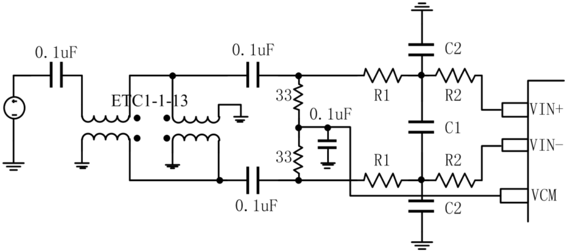
图 14 差分双巴伦输入配置
