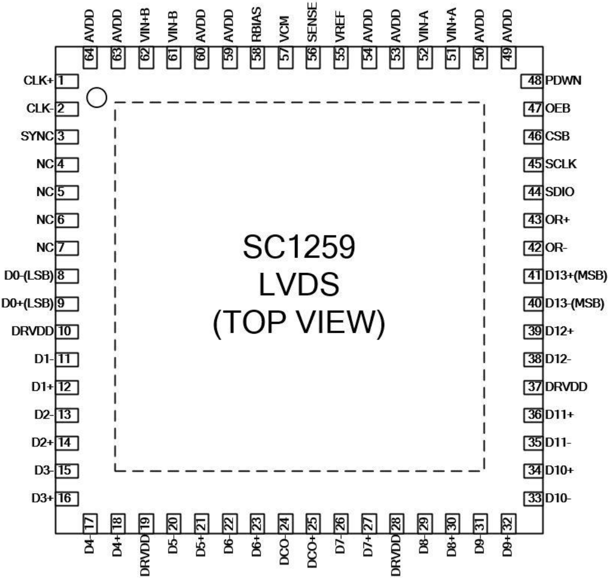
图 7 LVDS 管脚（焊盘）配置
