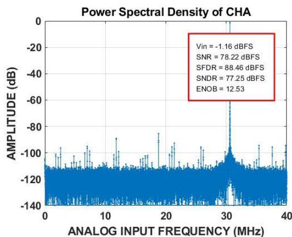
图 12 单音 FFT(fin = 30.5MHz@80MSPS)
