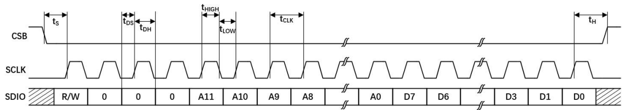
图 5 串行端口接口时序
