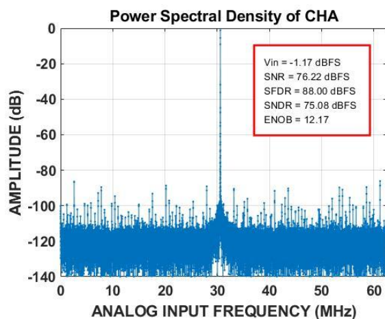
图 8 单音 FFT(fin = 30.5MHz@125MSPS)
