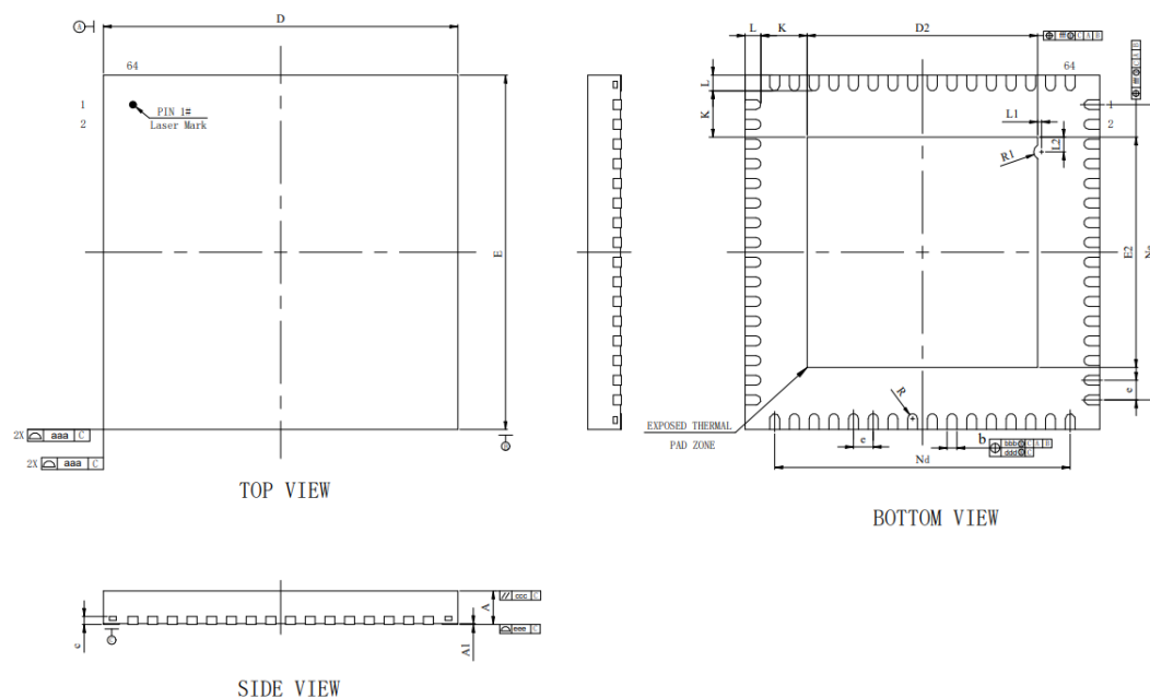
图 16 64 脚 QFN 封装尺寸图
