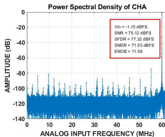
图 9 单音 FFT(fin = 60MHz@125MSPS)
