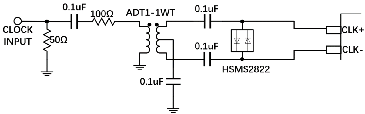
图 15 时钟输入配置
