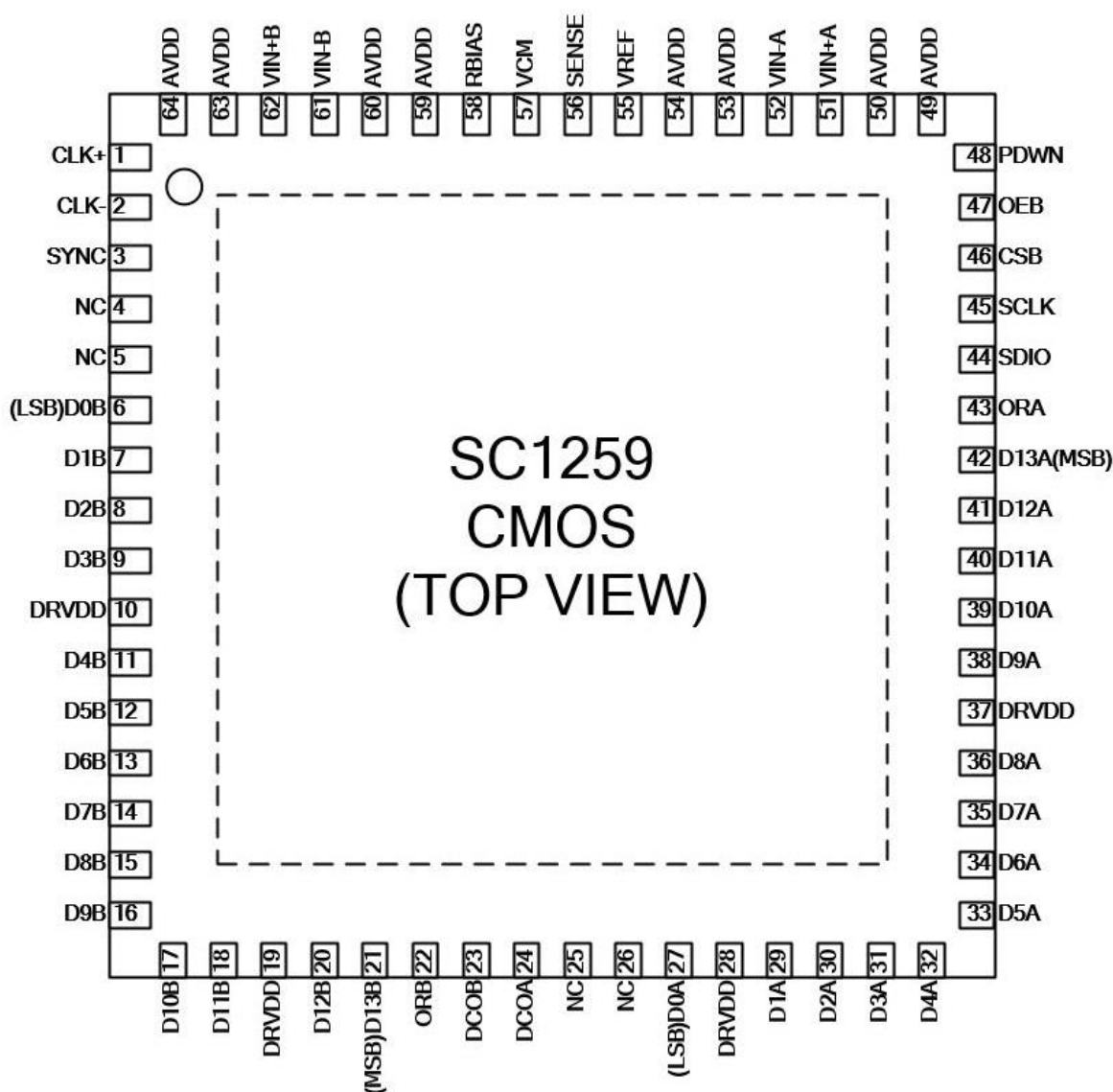
图 6 管脚（焊盘）配置
