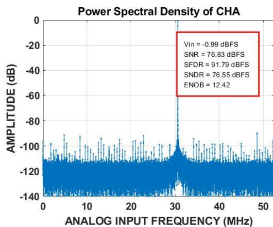
图 10 单音 FFT(fin = 30.5MHz@105MSPS)
