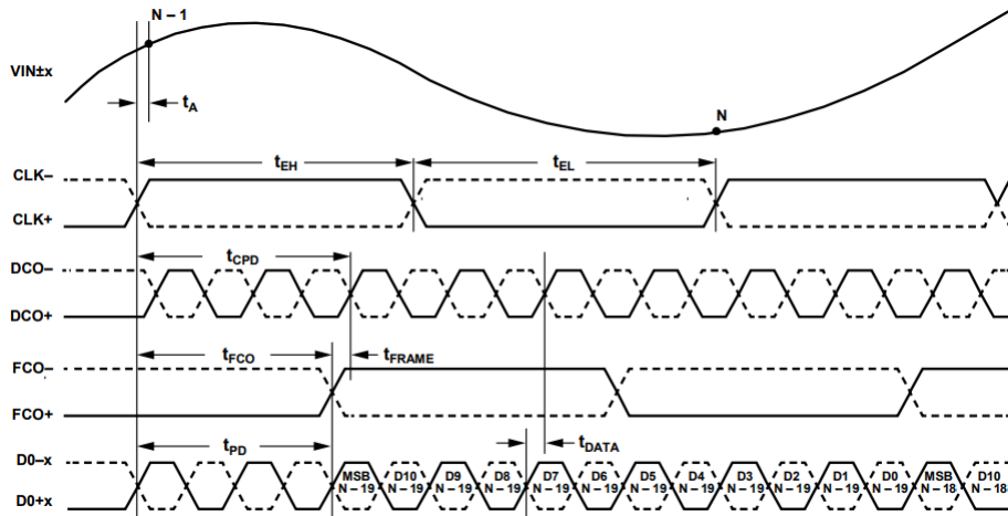
图 7 12-Bit DDR, One-Lane, 1×Frame 工作时序图
