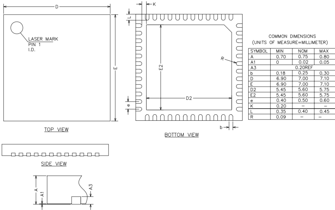
图 21 48 脚 QFN 封装尺寸图
