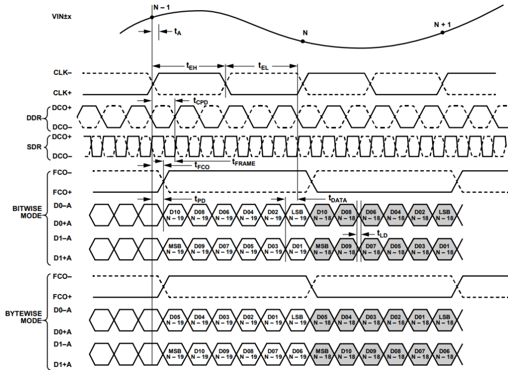
图 5 12-Bit DDR/SDR, Two-Lane, 2×Frame 工作时序图
