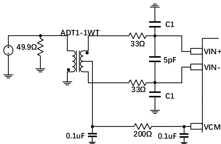
图 19 差动变压器耦合输入配置
